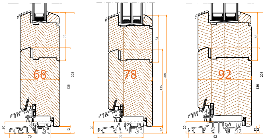
PROFIL 68 - ECOLINE
